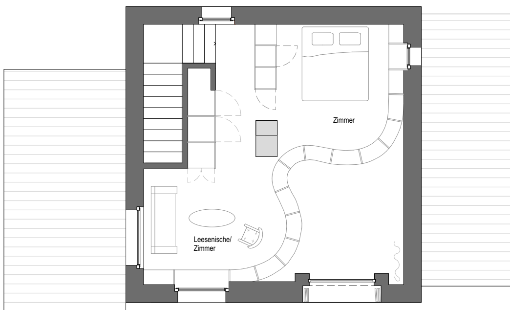
Obergeschoss 1:100
