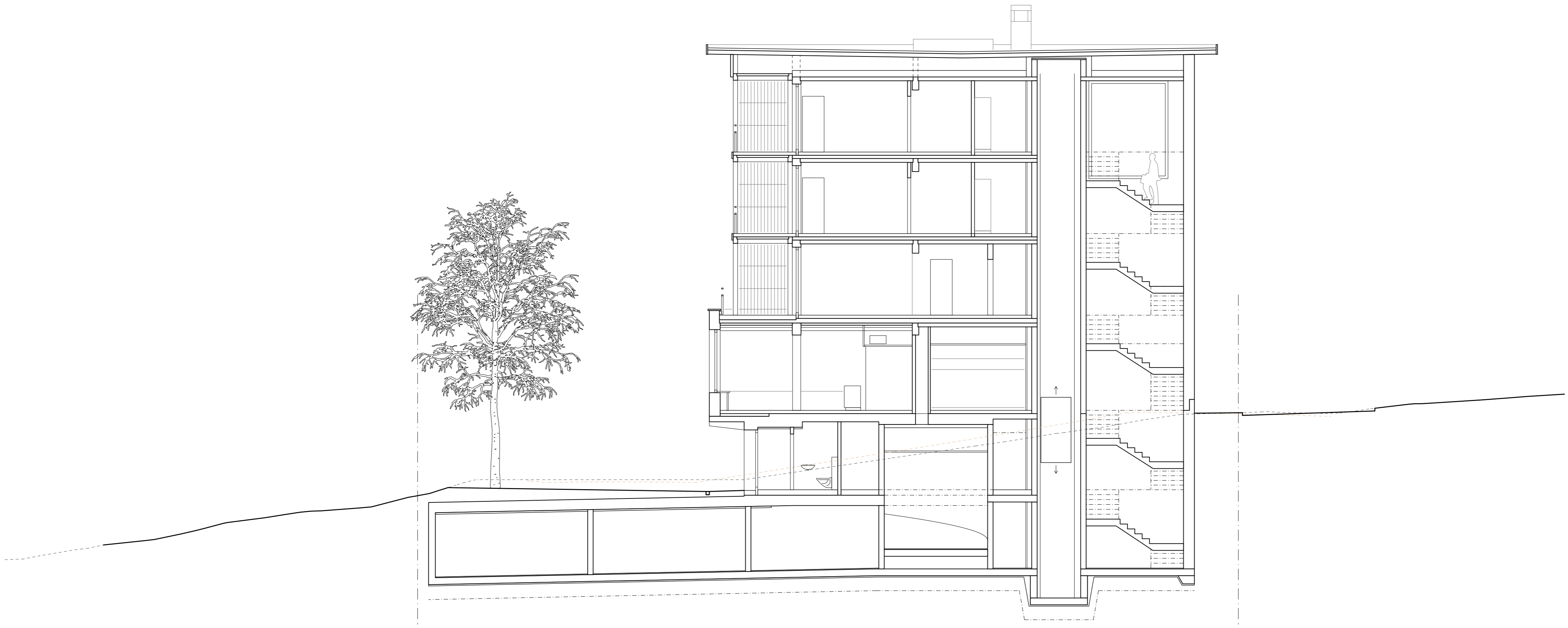
Querschnitt 1:200
